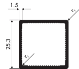
91030 0,36 kg/m obwód 99,48 mm
