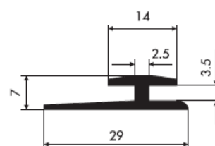
73006 0,19 kg/m obwód 178,46 mm
