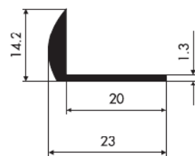
72011 0,16 kg/m obwód 70,32 mm
