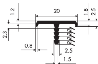
72009 0,12 kg/m obwód 67,84 mm
