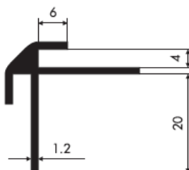
73005 0,24 kg/m obwód 123,61 mm
