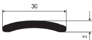
72008 0,23 kg/m obwód 64,79 mm
