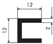
74003 0,18 kg/m obwód 66,28 mm
