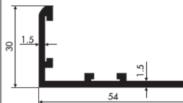
20515 0,42 kg/m obwód 200,95 mm
