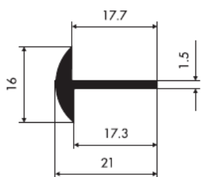
72012 0,18 kg/m obwód 67,16 mm
