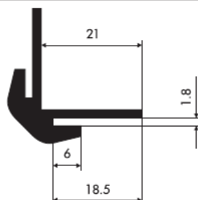
73002 0,30 kg/m obwód 120,86 mm
