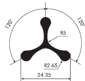
72021 0,33 kg/m obwód 88,13 mm
