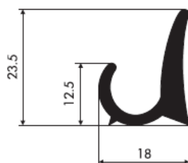
72013 0,33 kg/m obwód 95,35 mm
