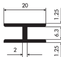
74006 0,17 kg/m obwód 91,20 mm
